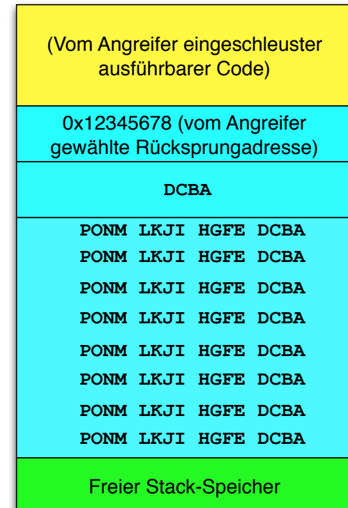
Stack bei Buffer Overflow
